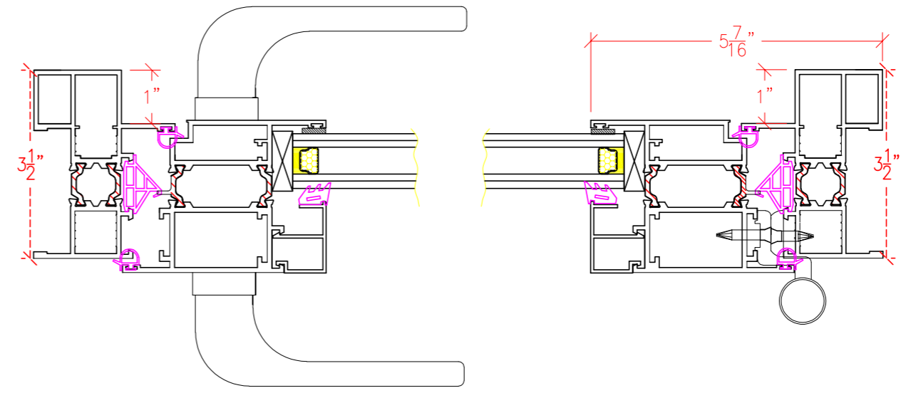
#2 Lock Jamb
